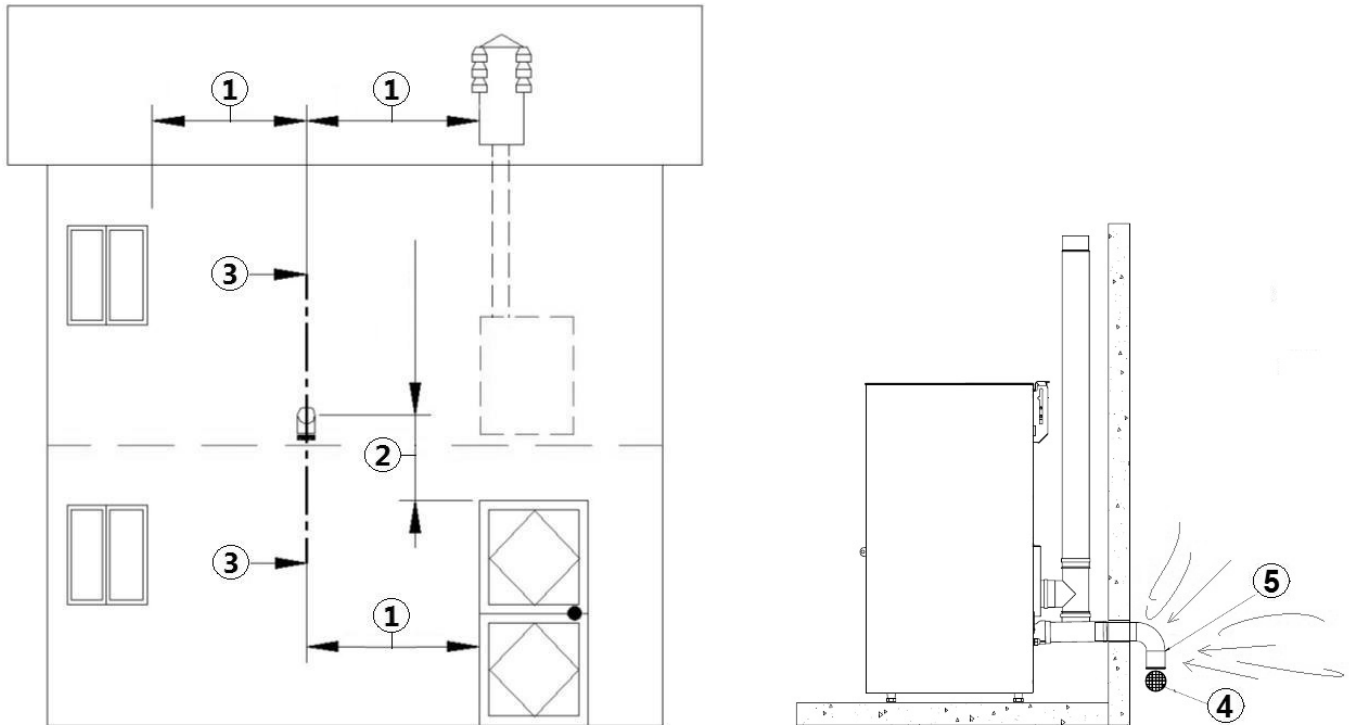
Fig. 11 - Luchtinlaat voor installatie met hermetisch gesloten kamer
