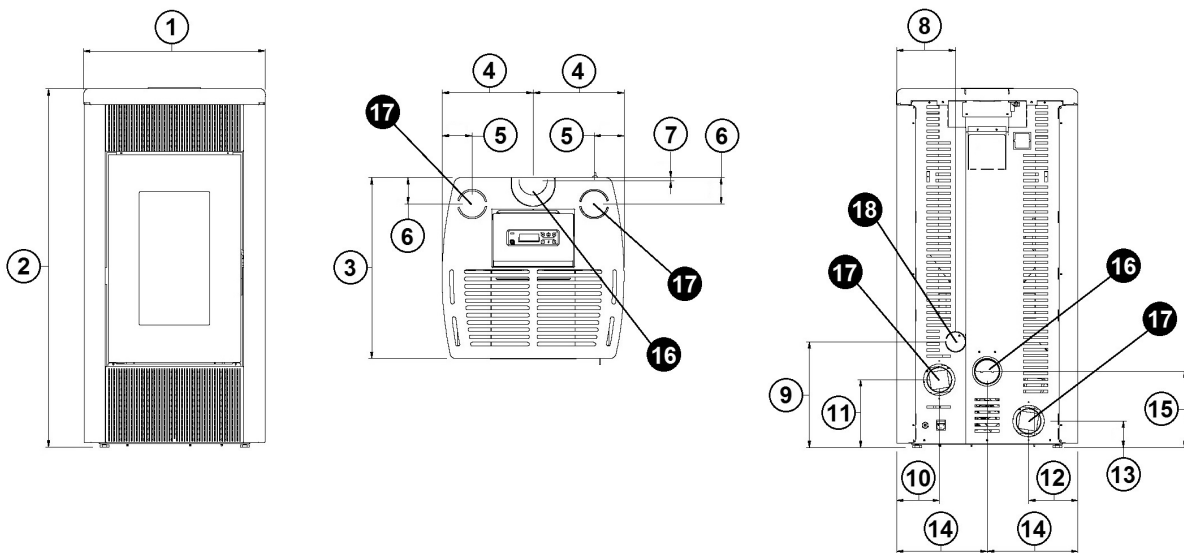
Fig. 14 - Algemene afmetingen: Duke 12/14 Airtight
