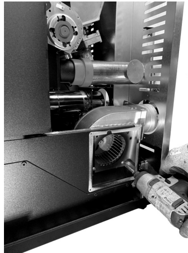
Fig. 49 - Bevestiging van de buis
