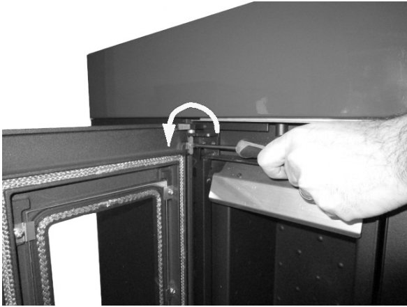
Fig. 17 - Verwijdering van de schroeven
