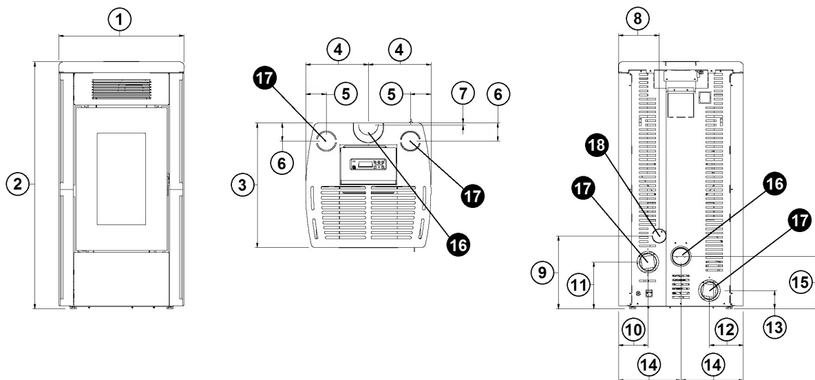
Fig. 13 - Algemene afmetingen: Atena³ Plus 12/14
