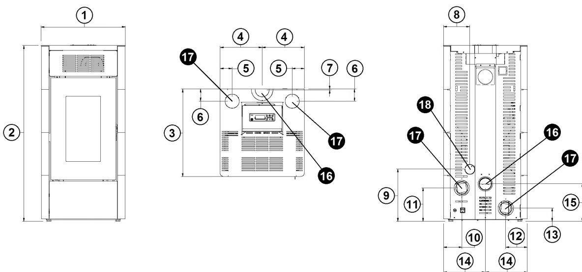
Fig. 15 - Algemene afmetingen: Saba 12/14
