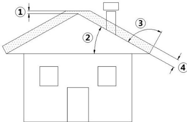
Fig. 3 - Schuin dak
