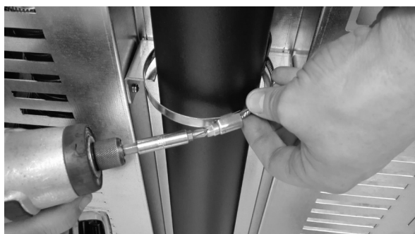
Fig. 44 - Blokkeer met klem
