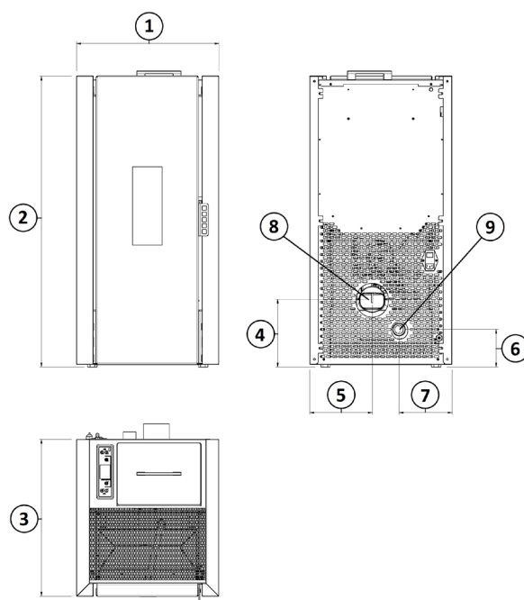
Fig. 13 - Algemene afmetingen: FREE/LUNA
