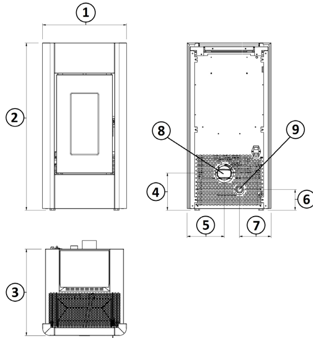
Fig. 14 - Algemene afmetingen: SWEET
