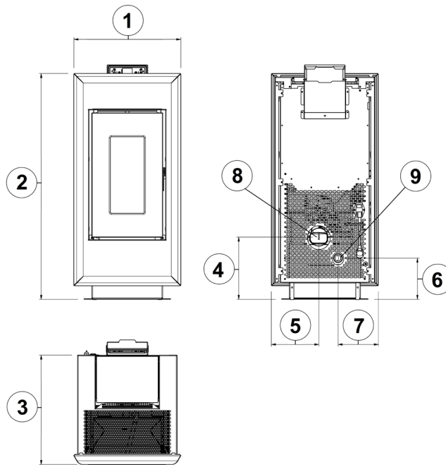
Fig. 17 - Algemene afmetingen: ELAN evo
