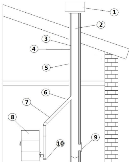
Fig. 6 - Onderdelen van de schoorsteen
