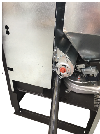
Fig. 50 - Reiniging omgevingsventilator
