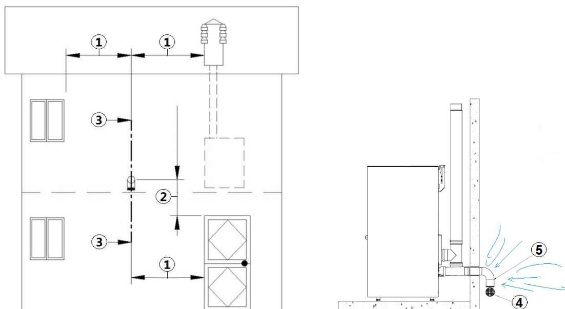
Fig. 8 - Luchtinlaat voor installatie
