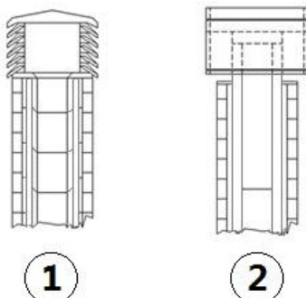
Fig. 5 - Windbestendige schoorsteenpotten
