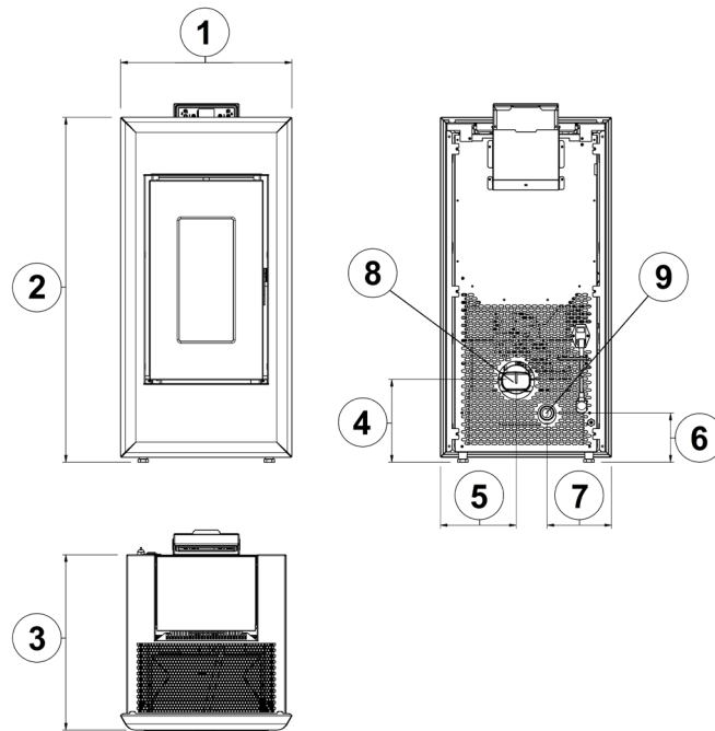
Fig. 15 - Algemene afmetingen: MIKA evo
