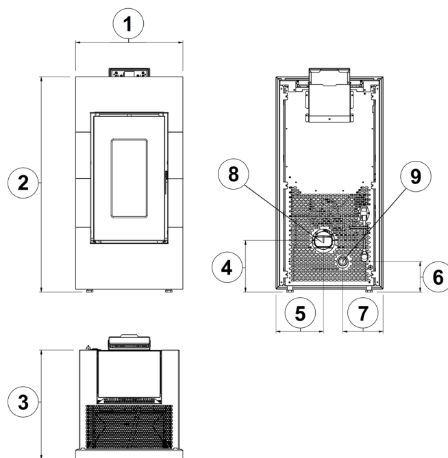
Fig. 16 - Algemene afmetingen: KAMI evo
