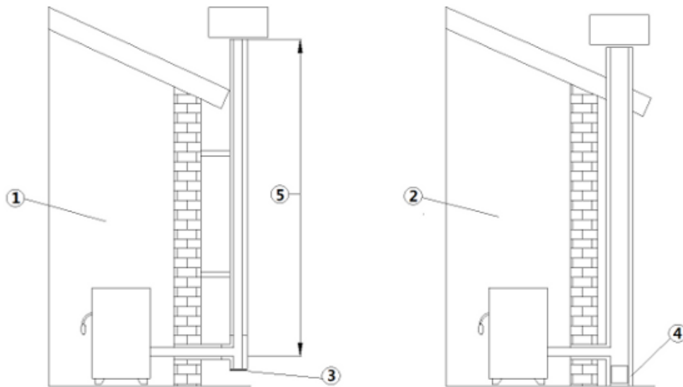
Fig. 2 - Rookkanalen
