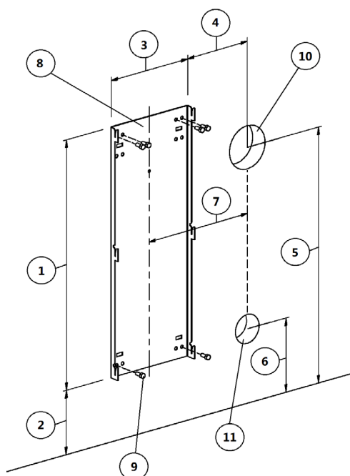
Fig. 19 - Bevestiging op niet ontvlambare muren
