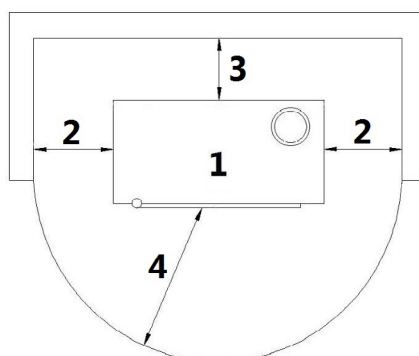
Fig. 15 - Algemene installatie met voetstuk
