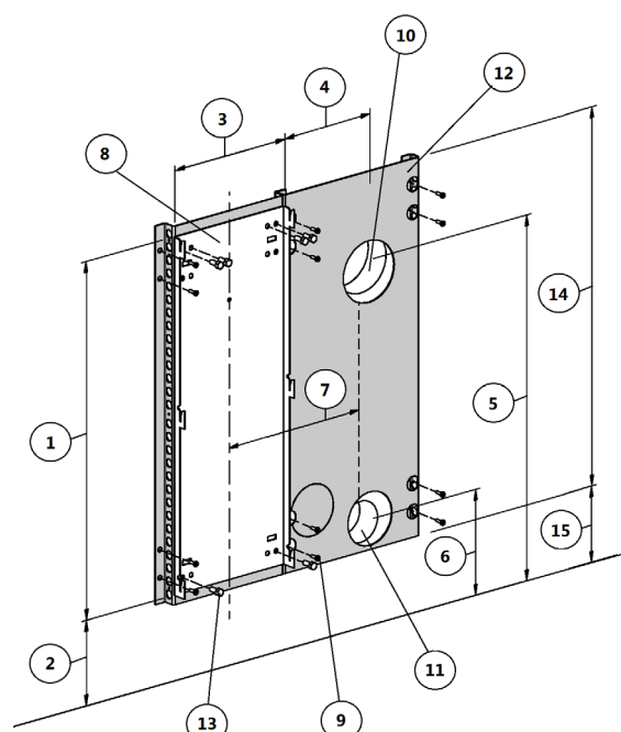
Fig. 20 - Bevestiging tegen een niet ontvlambare muur
