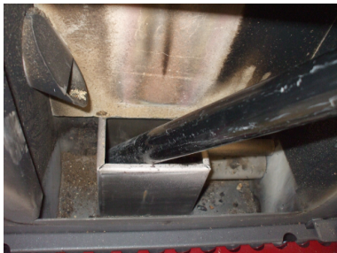
Fig. 30 - Reiniging ruimte vuurpot
