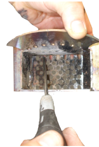
Fig. 29 - Reiniging vuurpot
