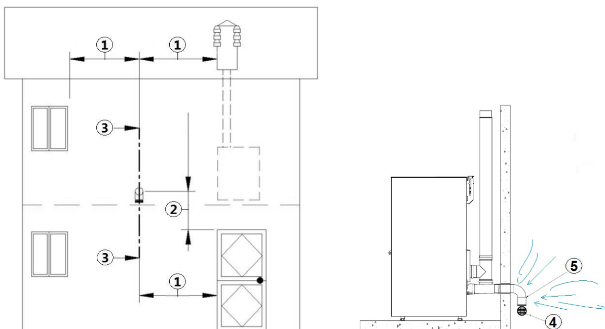
Fig. 7 - Luchtinlaat voor installatie met hermetisch gesloten kamer
