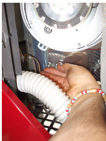
Fig. 34 - Fume chamber
