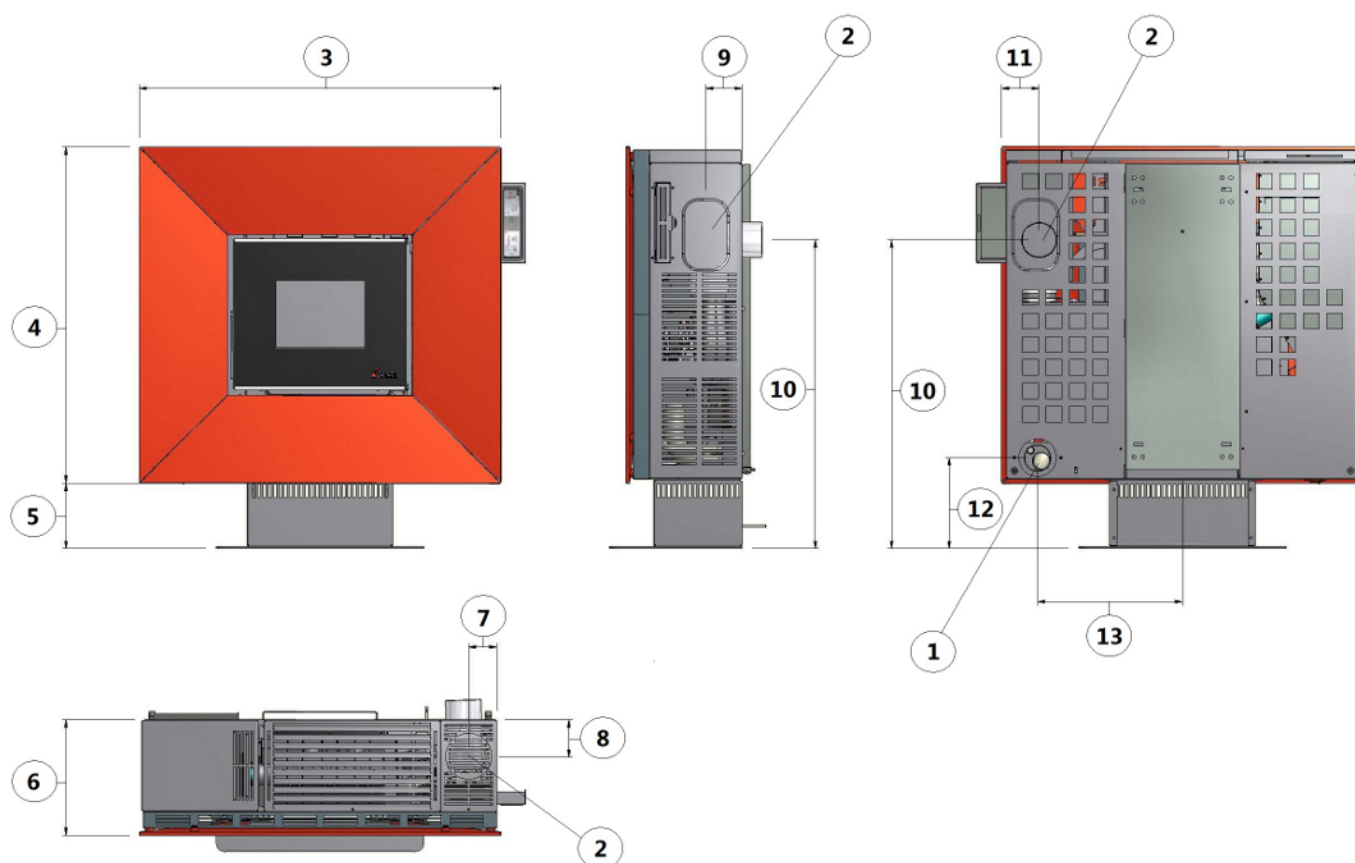
Fig. 14 - Algemene afmetingen
