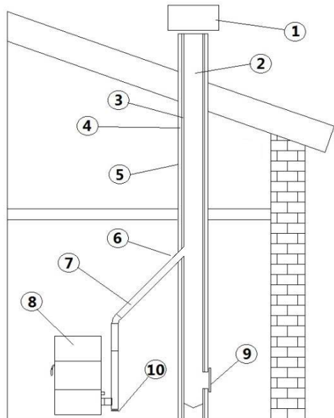
Fig. 6 - Onderdelen van de schoorsteen
