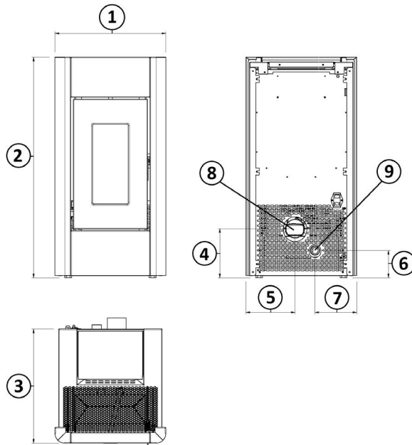
Fig. 17 - Algemene afmetingen: SWEET³
