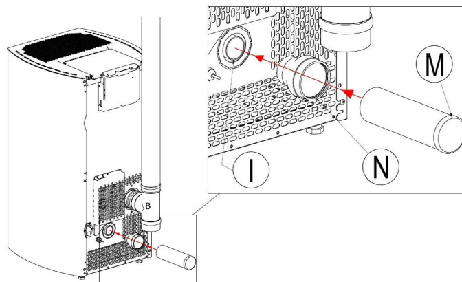
Fig. 9 - Verbindingen
