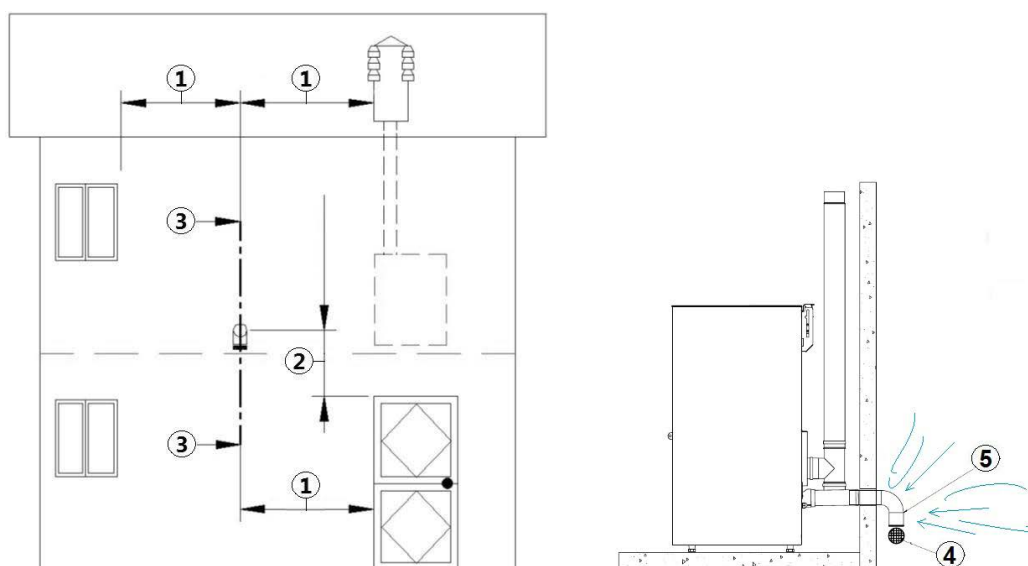
Fig. 8 - Luchtinlaat voor installatie met hermetisch gesloten kamer
