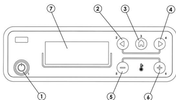
Fig. 33 - Display bedieningspaneel
