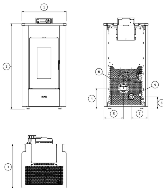
Fig. 18 - Algemene afmetingen: SHARP
