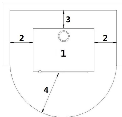
Fig. 19 - Algemene installatie
