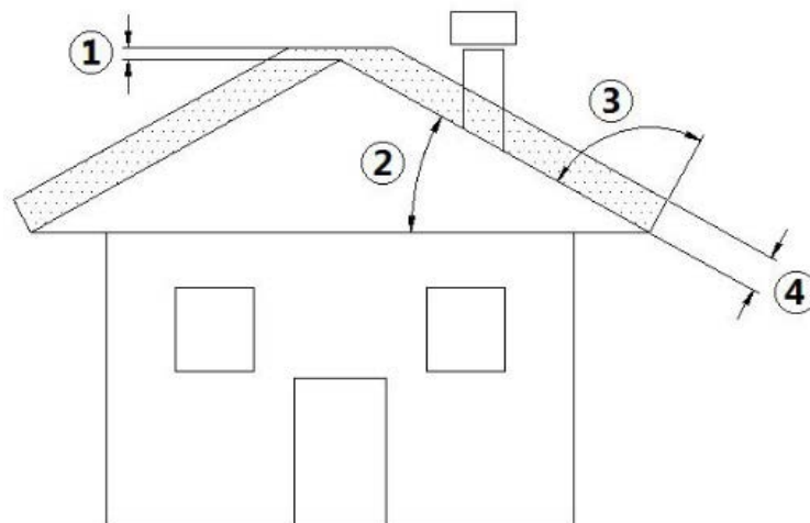
Fig. 3 - Schuin dak
