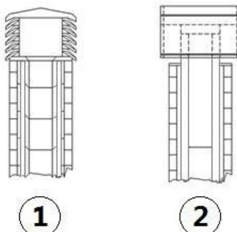
Fig. 5 - Windbestendige schoorsteenpotten
