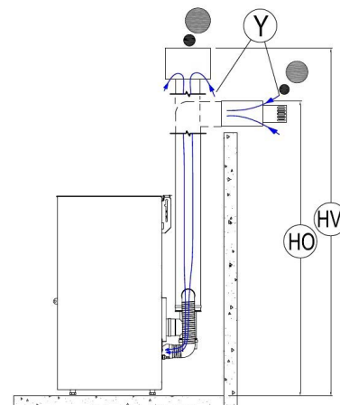
Fig. 12 - Verbindingen schoorsteenpijp
