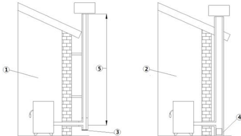
Fig. 2 - Rookkanalen
