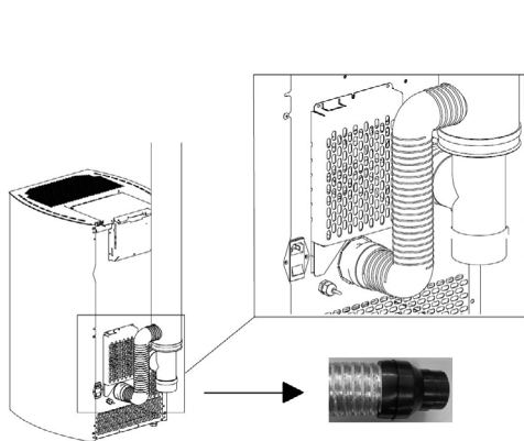
Fig. 10 - Flexibele buis
