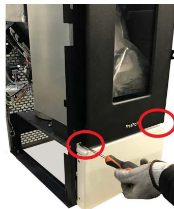
Fig. 21 - Bevestig het voorpaneel
