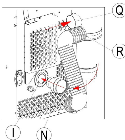
Fig. 11 - Verbindingen
