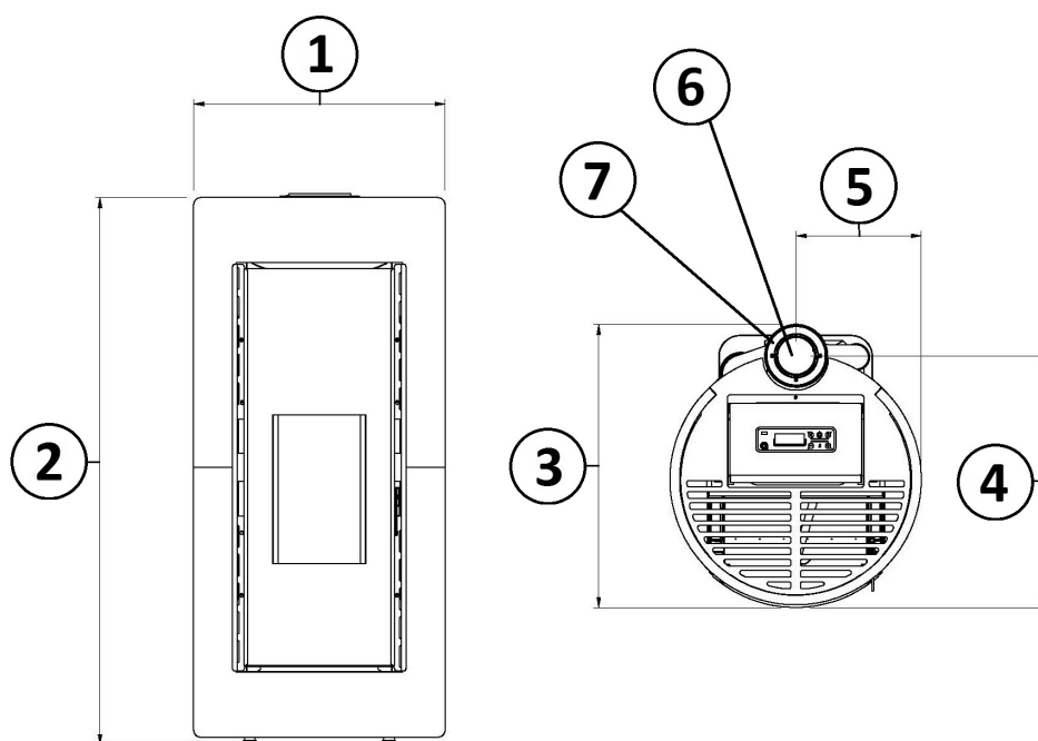
Fig. 33 - Dimensions générales: Shell P Up
