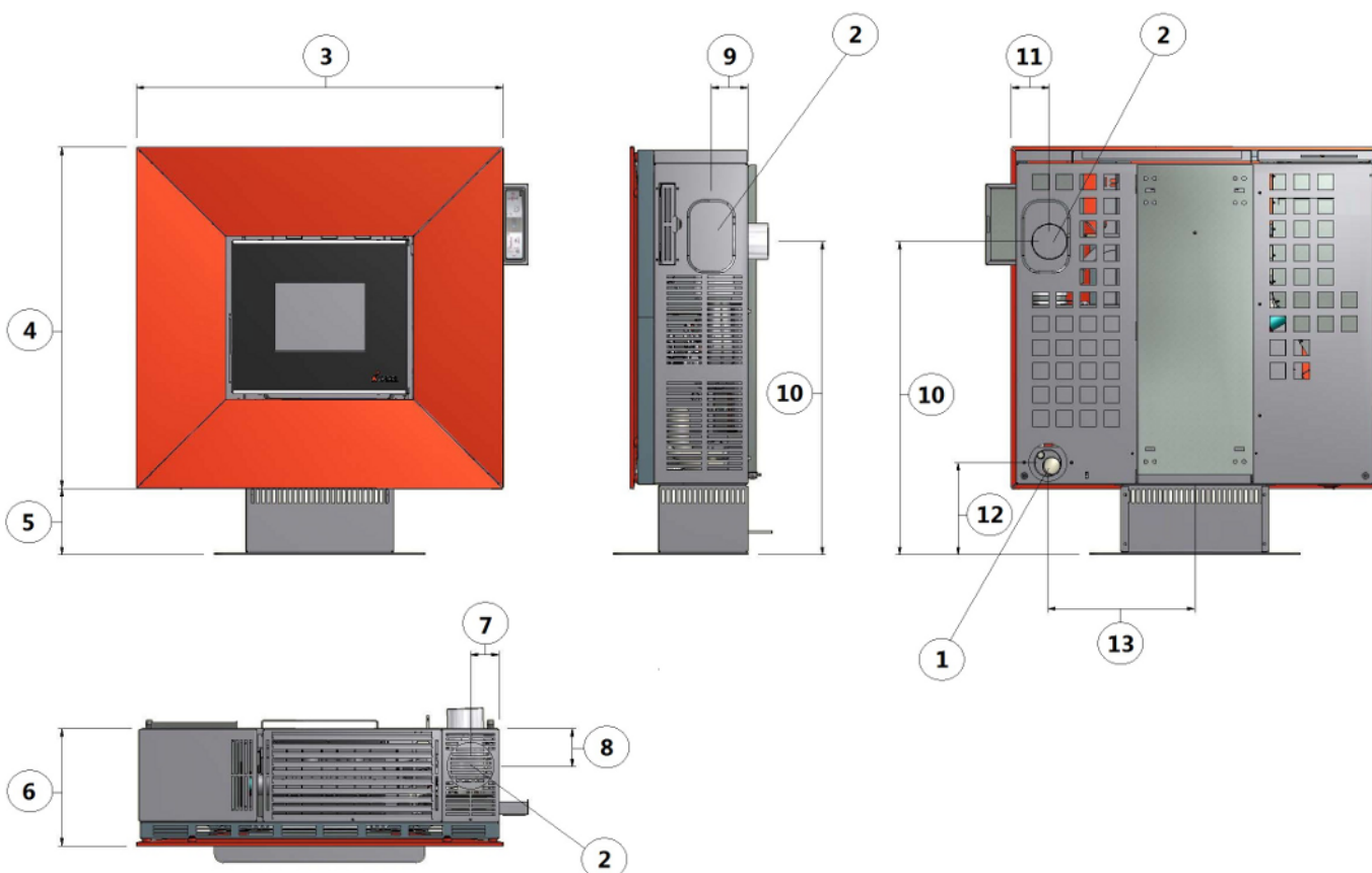
Fig. 14 - Dimensioni generali
