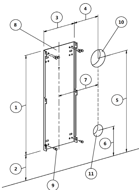
Fig. 19 - Fissaggio su parete non infiammabili
