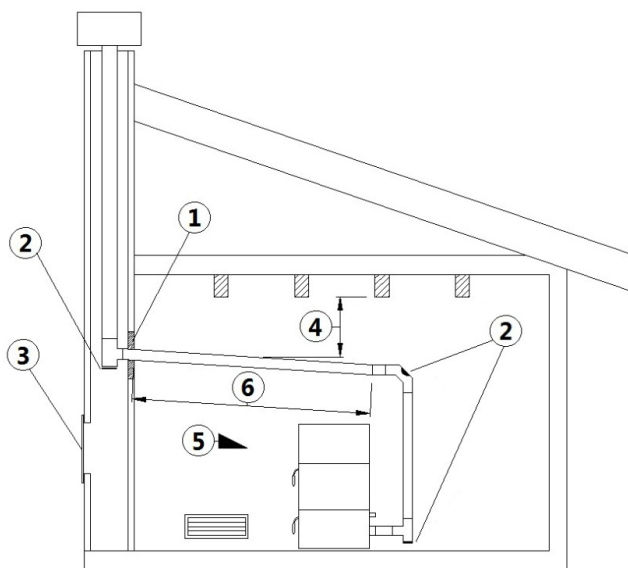
Fig. 12 - Esempio 2
