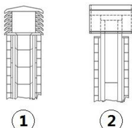
Fig. 4 - Comignoli antivento
