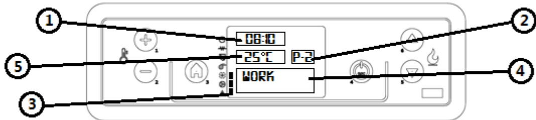
Fig. 23 - Tableau de contrôle LCD
