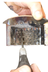
Fig. 29 - Pulizia braciere
