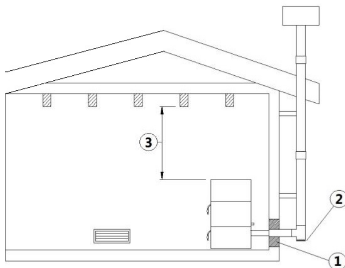
Fig. 13 - Esempio 3
