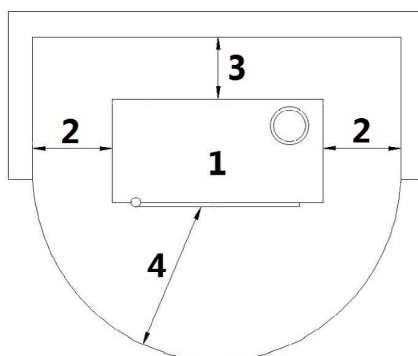
Fig. 15 - Installazione generica con piedistallo
