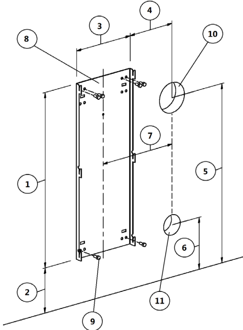
Fig. 19 - Fixation au mur non inflammable
