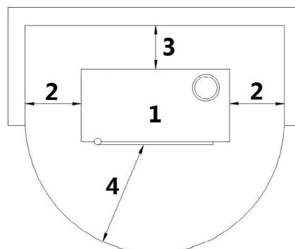
Fig. 15 - Installation générique avec piédestal
