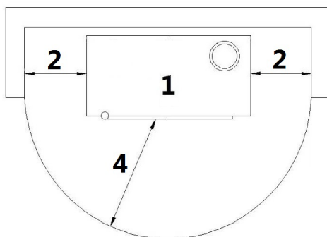
Fig. 18 - Installazione a parete
