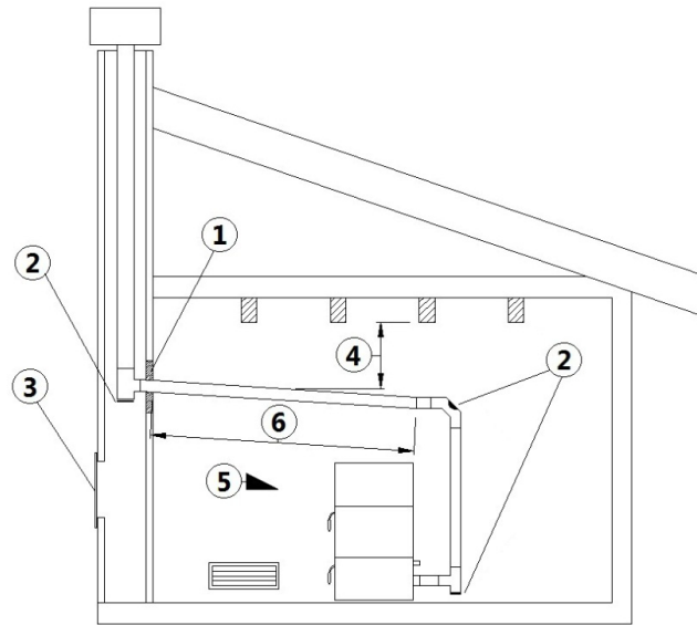
Fig. 12 - Exemple 2
