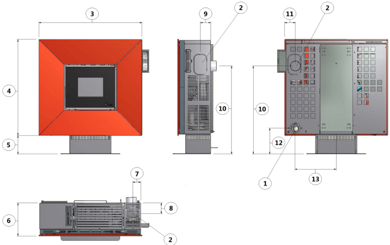
Fig. 14 - Dimensions générales
