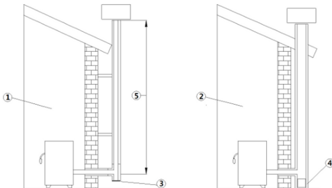
Fig. 1 - Canne fumarie
