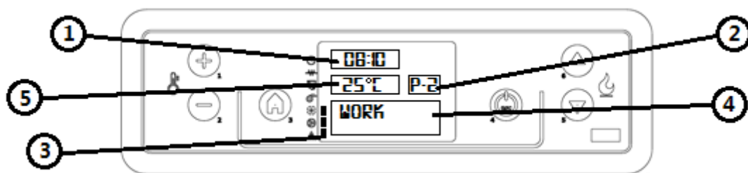
Fig. 23 - Display di controllo LCD
