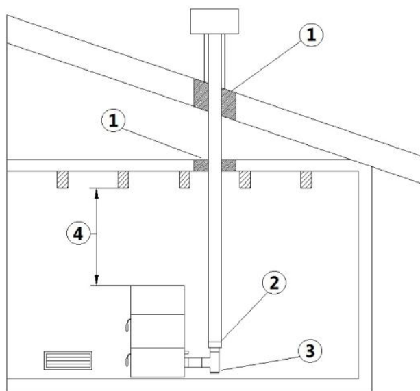
Fig. 11 - Esempio 1
