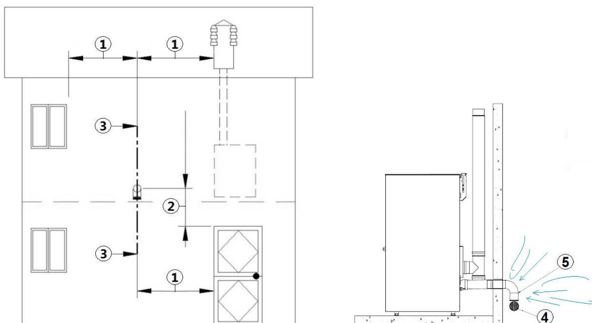
Fig. 7 - Presa d'aria per installazione a camera stagna
