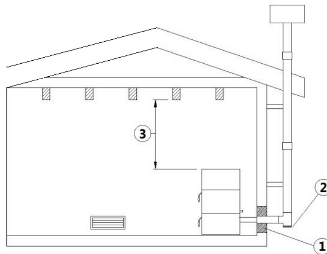
Fig. 13 - Exemple 3
