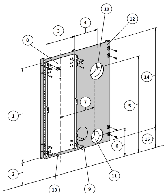
Fig. 20 - Fissaggio su parete infiammabili
