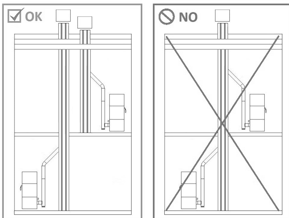
Fig. 10 - Exemples des installations correctes
