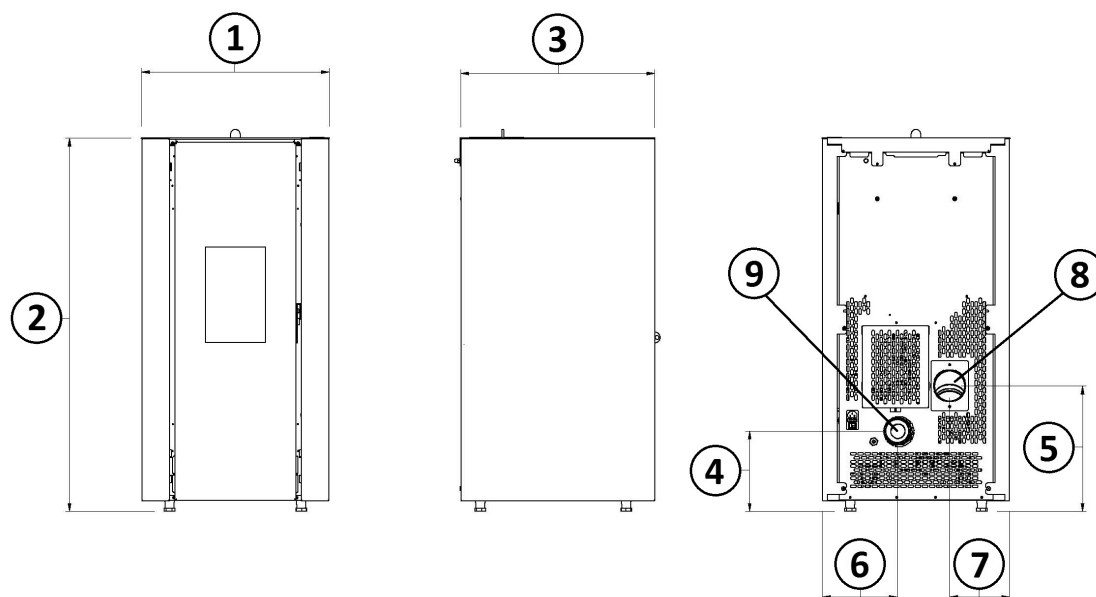
Fig. 17 - Dimensions générales: ELANE
