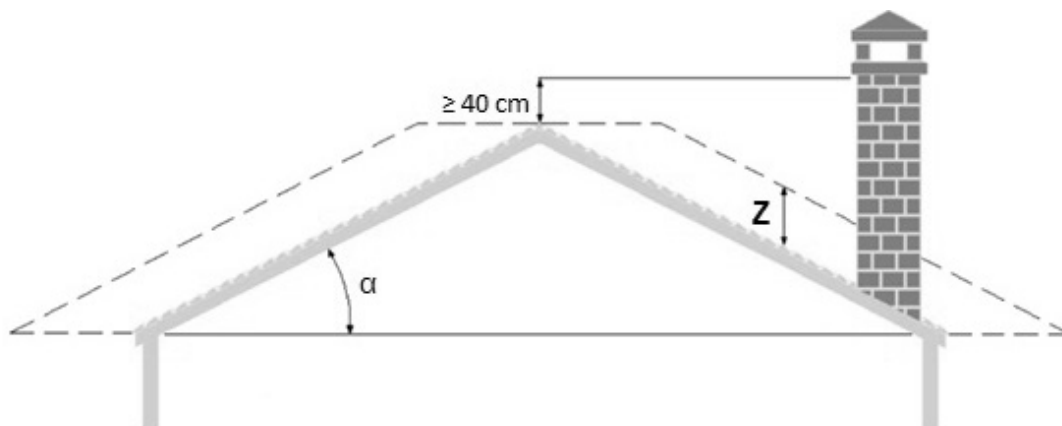
Fig. 6 - Zones de reflux
