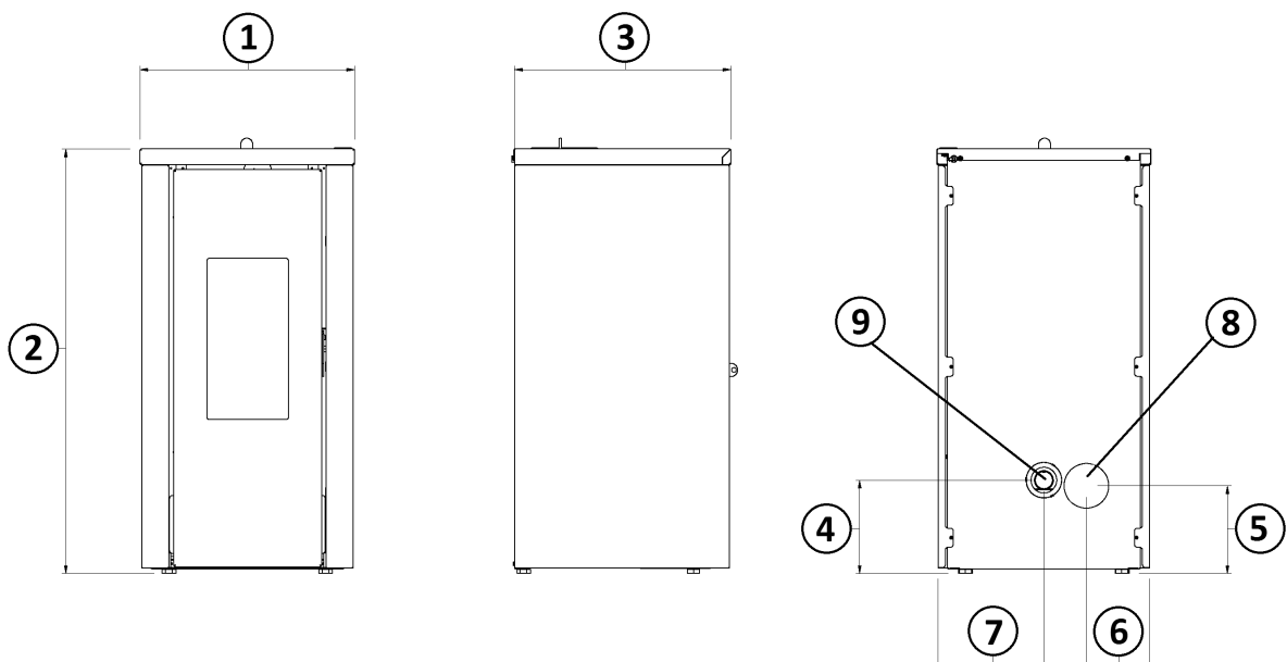
Fig. 15 - Dimensions générales: VERA
