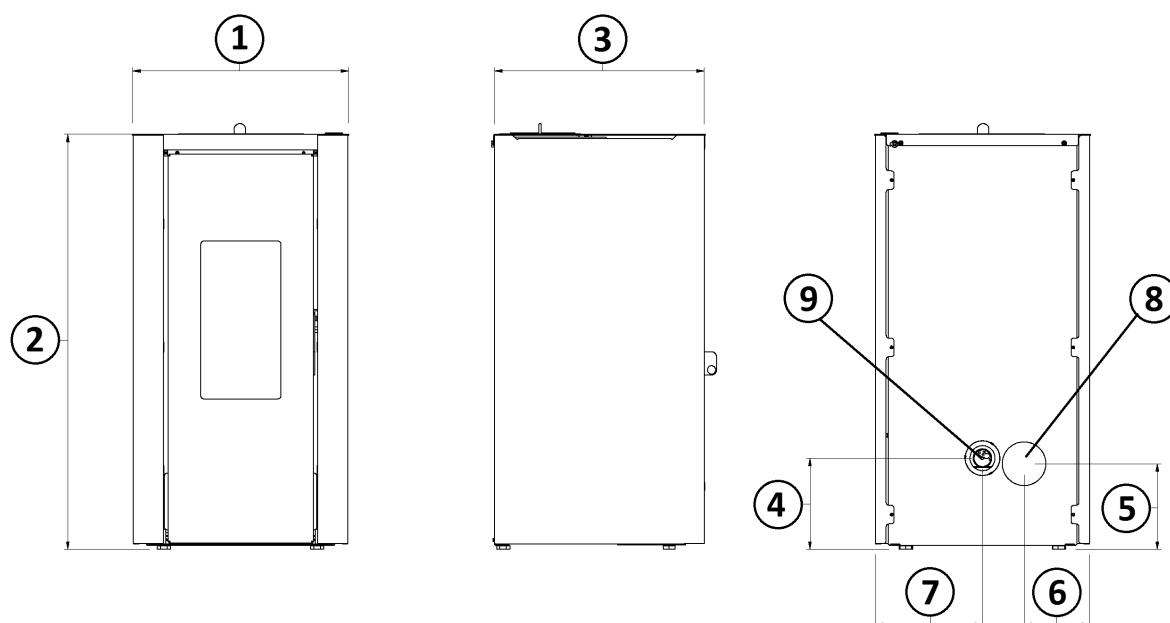
Fig. 14 - Dimensions générales: INDIGO AT
