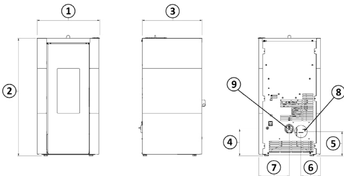
Fig. 16 - Dimensions générales: TALAS 3
