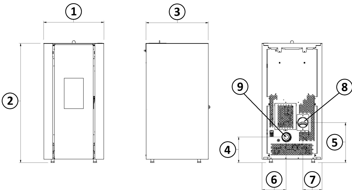
Fig. 16 - Algemene afmetingen: ELANE
