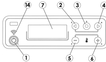
Fig. 9 - Bedieningspaneel (wi-fi)
