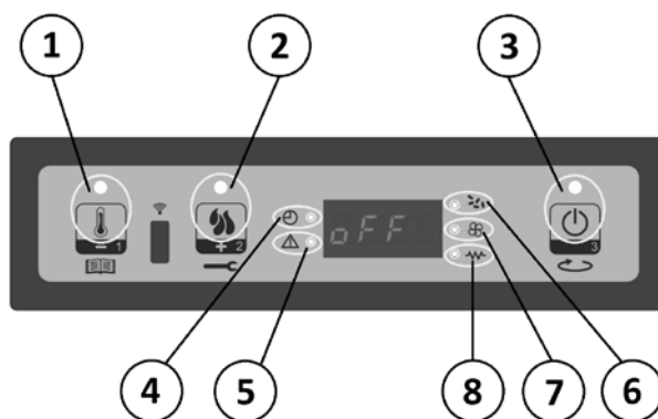
Fig. 5 - Display: ingeschakelde leds
