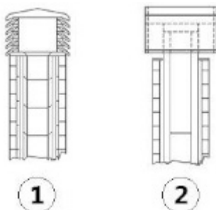
Fig. 5 - Windbestendige schoorsteenpotten
