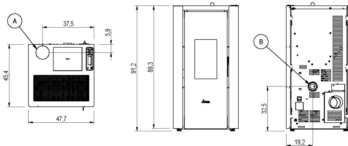
Fig. 15 - Algemene afmetingen: CRISTAL3 7.0 UP
