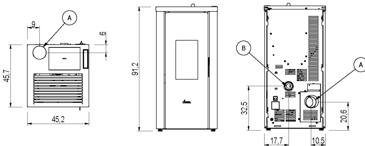
Fig. 14 - Algemene afmetingen:VERA 7.0 UP
