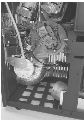
Fig. 41 - Installeer de flexibele buis
