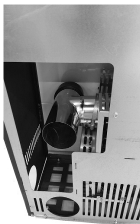
Fig. 50 - De afvoerbuis aansluiten
