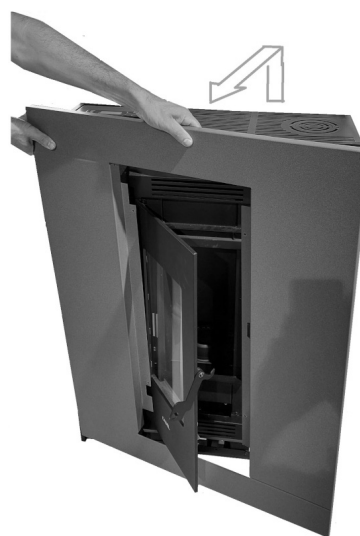
Fig. 20 - De lijst verwijderen
