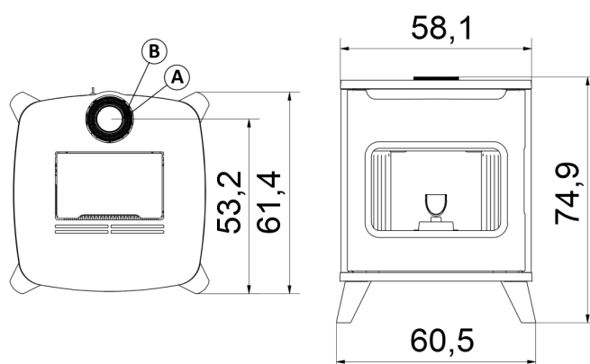
Fig. 13 - Algemene afmetingen: HUBLLOT 6 UP
