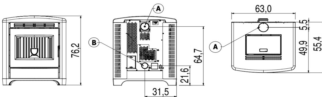
Fig. 12 - Algemene afmetingen: MAGRITTE 6
