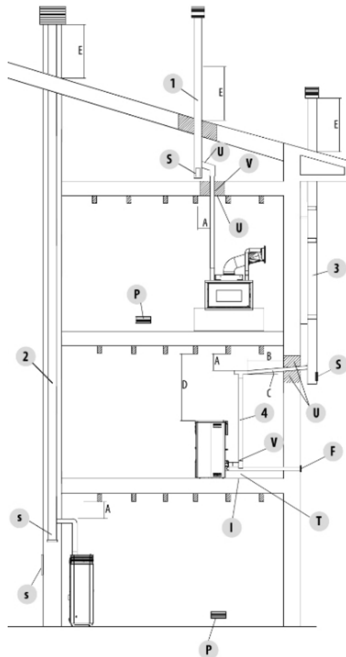
Fig. 10 - Rookkanaal
