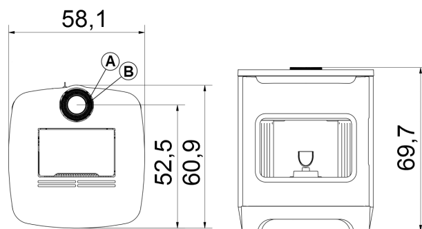
Fig. 14 - Algemene afmetingen: FLOS 6
