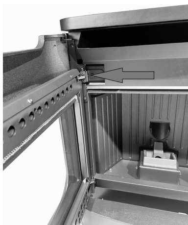
Fig. 17 - Deur afstellen
