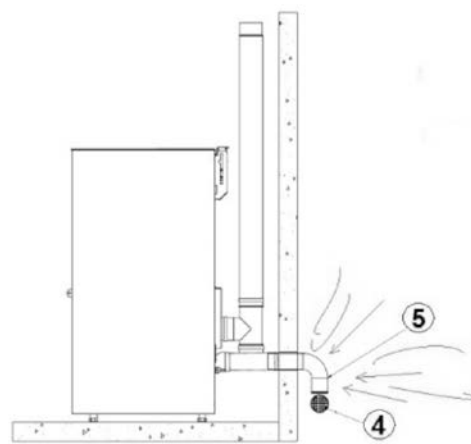
Fig. 8 - Luchtinlaat voor installatie met hermetisch gesloten kamer
