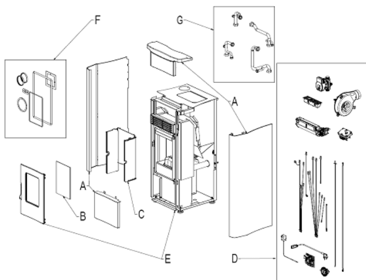
Fig. 1 - Dessin éclaté
