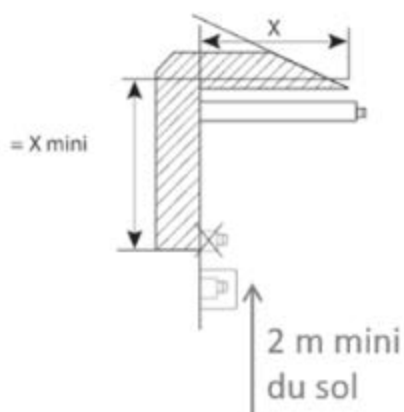
Fig. 17 - Rebord de toit
