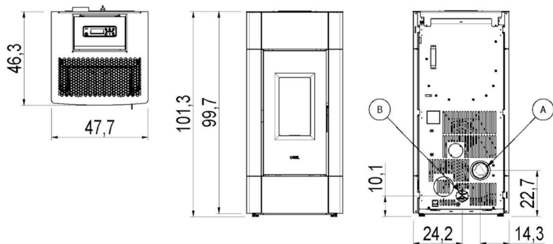
Fig. 24 - Dimensions générales: Cristal 9
