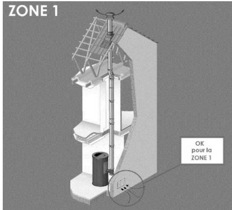
Fig. 18 - Installation possible pour tous les poêles (ZONE 1)
