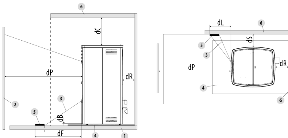
Fig. 23 - Distances de sécurité
