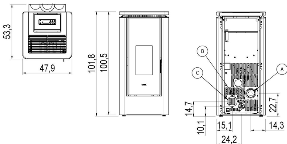
Fig. 26 - Dimensions générales: Icon Plus 9
