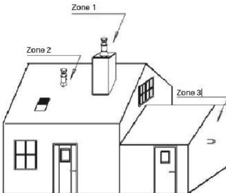
Fig. 15 - Définition des zones d'implantation
