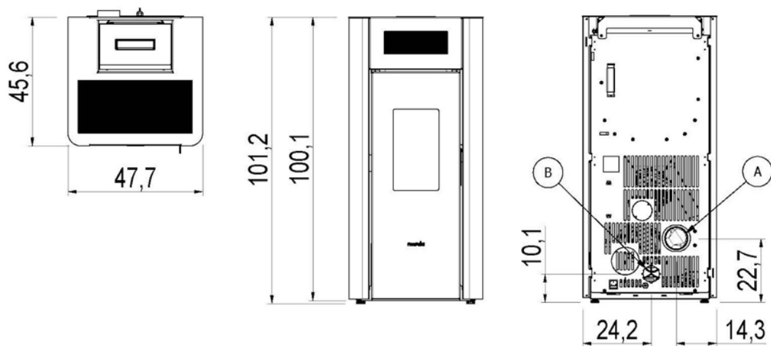
Fig. 27 - Dimensions générales: Amaranto 9
