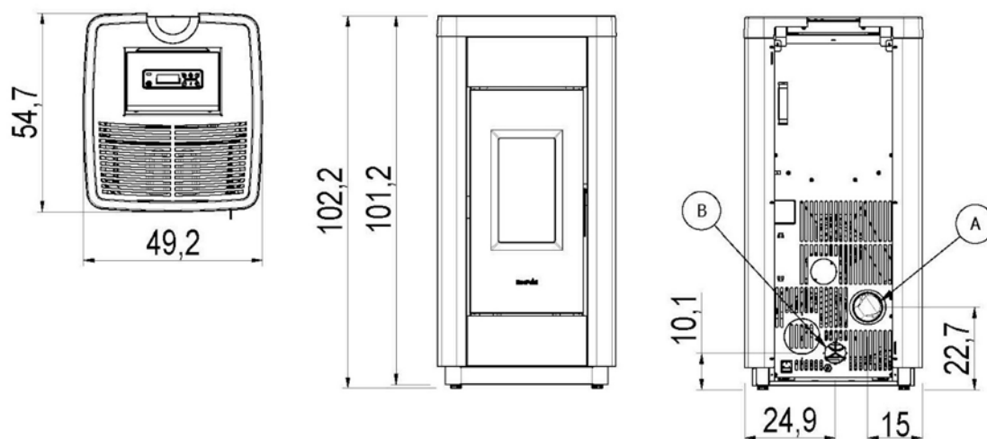
Fig. 28 - Dimensions générales: Life 9
