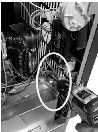
Fig. 69 - Extraire le tuyau flexible
