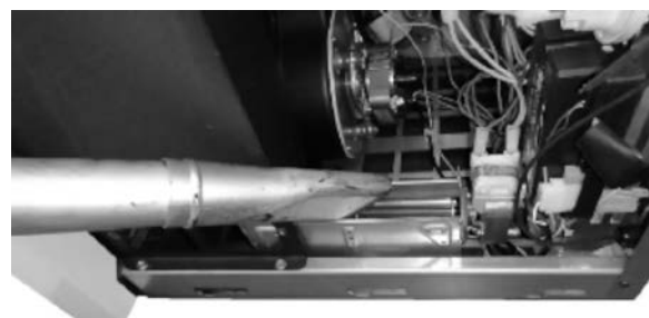
Fig. 90 - Nettoyage de le ventilateur ambiant (Mithos 3 Plus 12/14)
