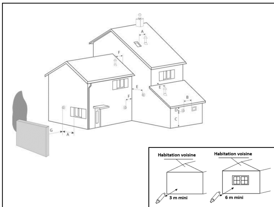
Fig. 16 - Position des terminaux
