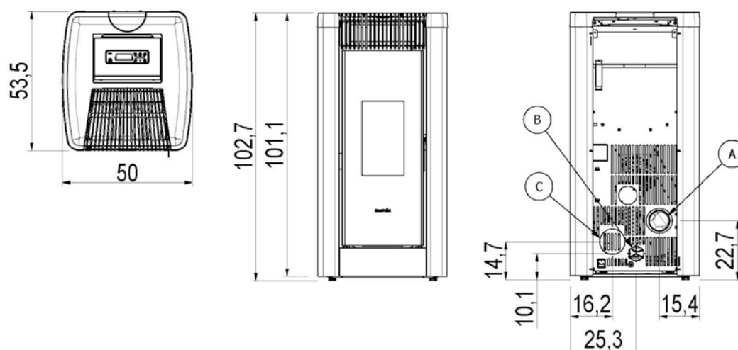
Fig. 29 - Dimensions générales: Steel 9
