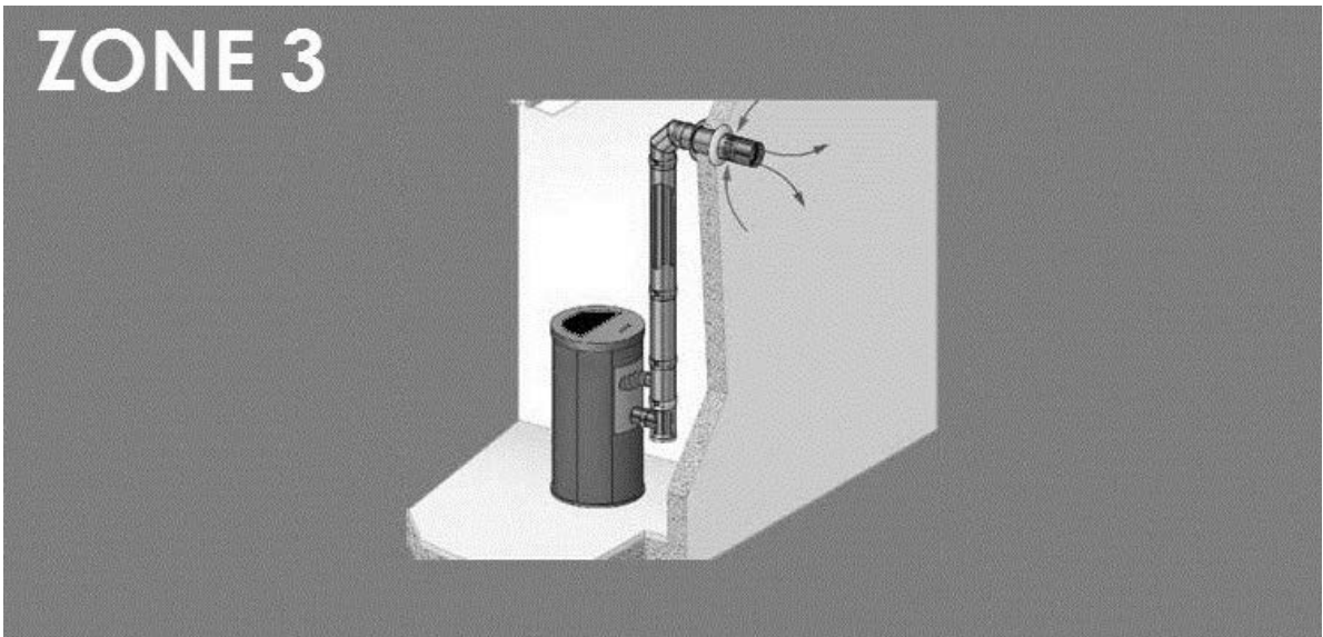
Fig. 20 - Schéma de principe du système concentrique avec terminal horizontal (ZONE 3)
