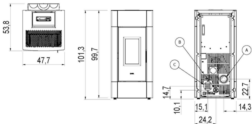
Fig. 25 - Dimensions générales: Cristal Plus 9
