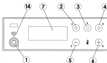
Fig. 7 - Bedieningspaneel (wi-fi)
