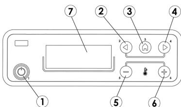
Fig. 6 - Bedieningspaneel
