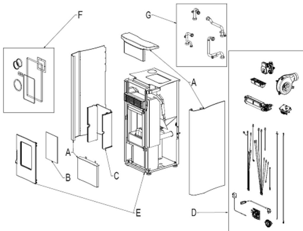
Fig. 1 - Geëxplodeerde tekening
