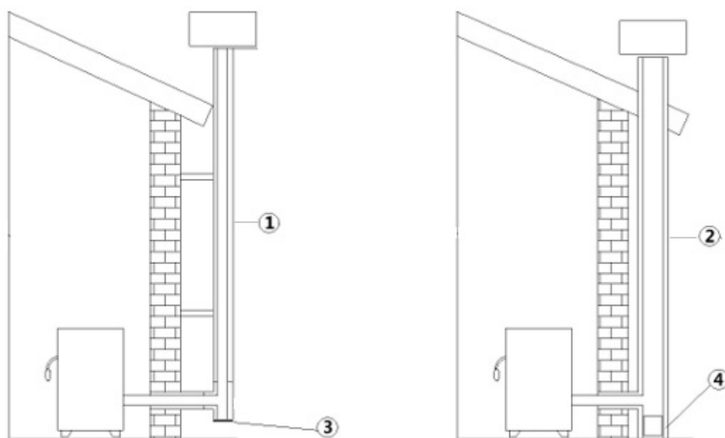
Fig. 3 - Rookkanalen
