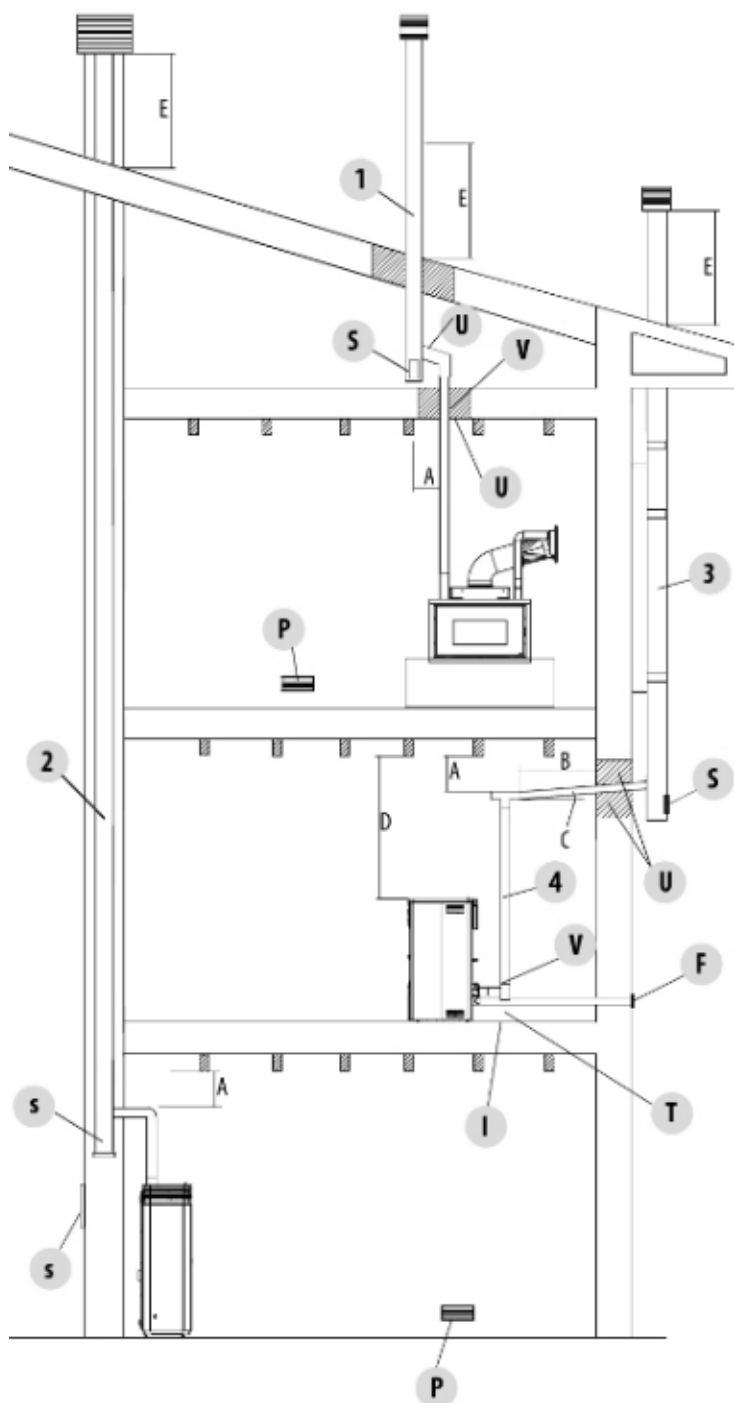
Fig. 10 - Rookkanaal
