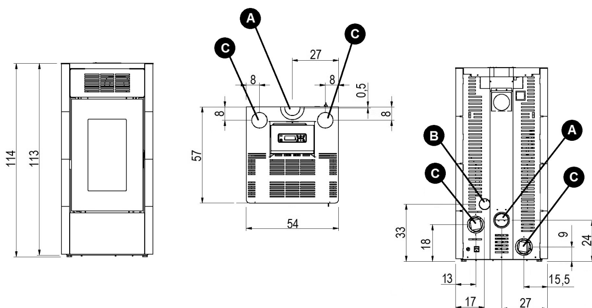
Fig. 12 - Algemene afmetingen: Saba 12/14
